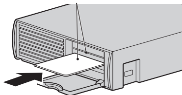
ICカード挿入口 (上段:C-CAS、下段:B-CAS)
